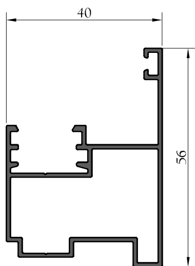
BUTEE POUR OUVRANT 02 VTX
