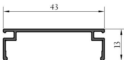
CAPOT DOUBLE VITRAGE
