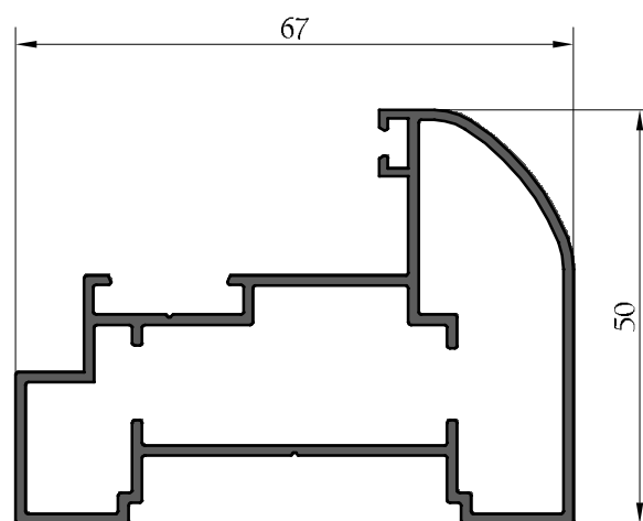
HUISSERIE
