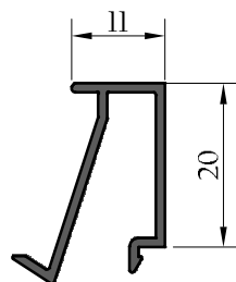
PARCLOSE DOUBLE VITRAGE
