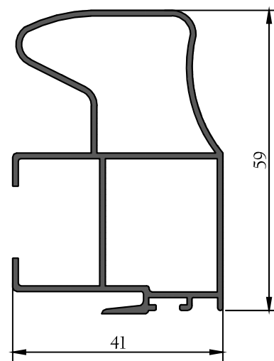
MONTANT CENTRAL AVEC RENFORT
