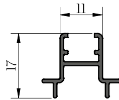
JONCTION 4 VANTAUX
