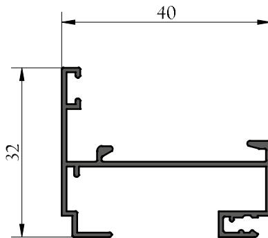
DORMANT SIMPLE
