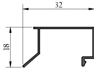
PARCLOSE
