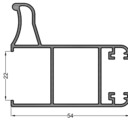
MONTANT LATERAL AVEC RENFORT
