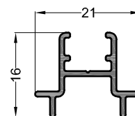
JONCTION 4 VANTAUX
