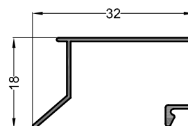
PARCLOSE
