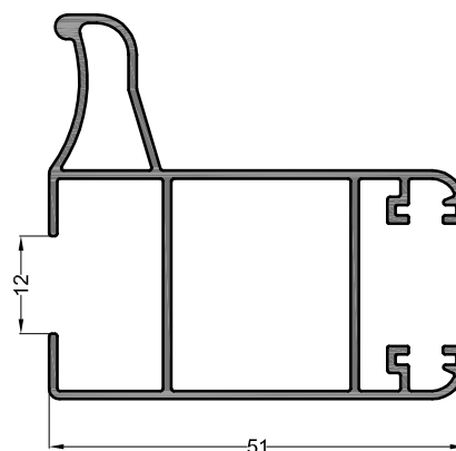
MONTANT LATERAL AVEC RENFORT
