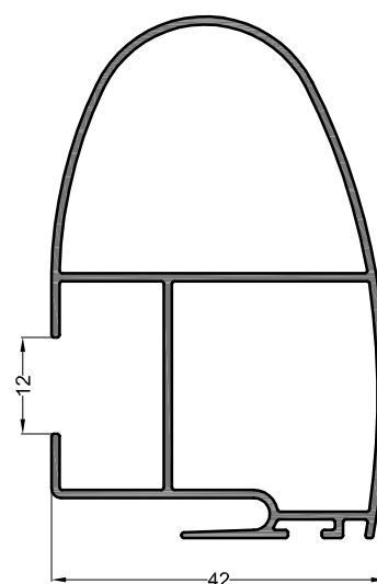
MONTANT CENTRAL AVEC RENFORT
