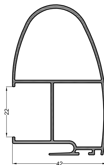
MONTANT CENTRAL AVEC RENFORT
