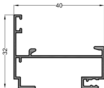
DORMANT SIMPLE
