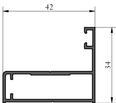
DORMANT VEC
