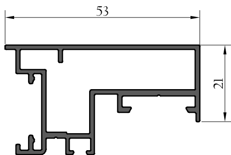
OUVRANT VEC
