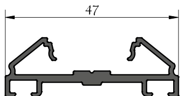
SERREUR 5037
