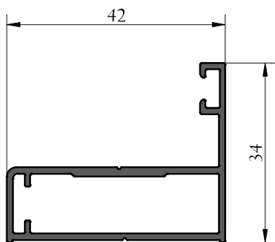
DORMANT VEC
