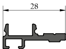
DEMI SERREUR 5029
