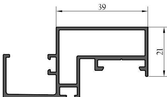
OUVRANT SEMI-VEC
