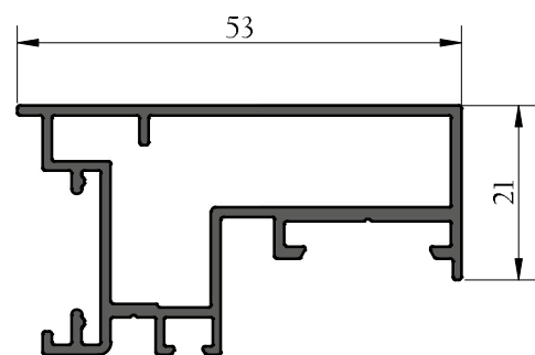
OUVRANT VEC
