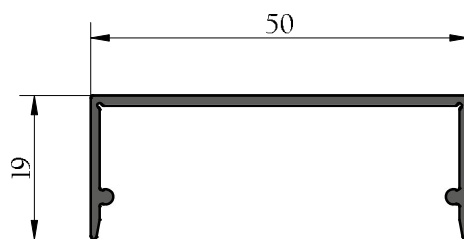
CAPOT PLAT 5026
