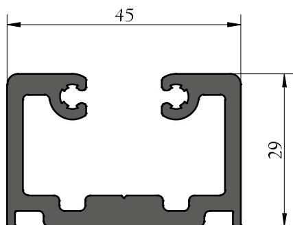
BLOC D'ASSEMBLAGE
